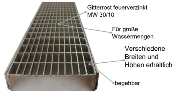
Abbildung 1: VOLFI Gitterrost in Kombination mit optional erhältlichen VOLFI Kastenrinnen.
