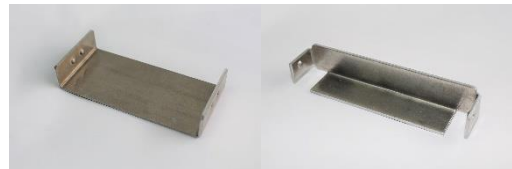
Abbildung 4: Verbinder f. KR-SL/KR-OL Abbildung 5: Abschlussplatte f. KR-SL/KR-OL
