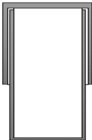
Abbildung 5: Kombination zweier Typen WD-C 17+37 -> Drainagehöhe ca. 39mm
