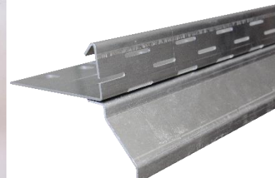
Abbildung 6+7: Abdeckprofil für Uniprofil VF mit vorgebohrten Löchern zum Anieten unter den Sichtschenkel des Profils.
