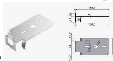
Abbildung 5: Abmessungen Stufenclip
