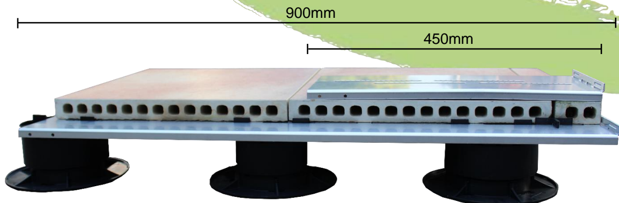
Abbildung 4: Die RWK lassen sich im gesamten VOLFI-System für die moderne Plattenverlegung kombinieren. Je länger die Konsole gewählt wird, desto mehr „überstehendes Gewicht“ kann diese aufnehmen.
