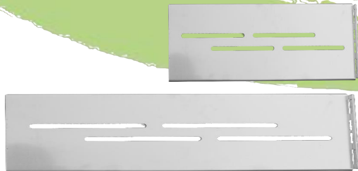
Abbildung 2: Die VOLFI – RWK wird in 2 verschiedenen Längen angeboten. Je länger, desto mehr Gewicht kann abgefangen, desto mehr Überstand kann überbückt werden.
