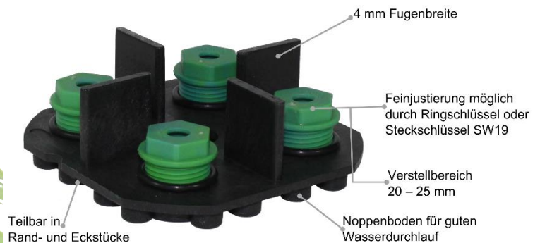
Abbildung 1: VOLFI-SKT-V Sechskant-Stelzlager
