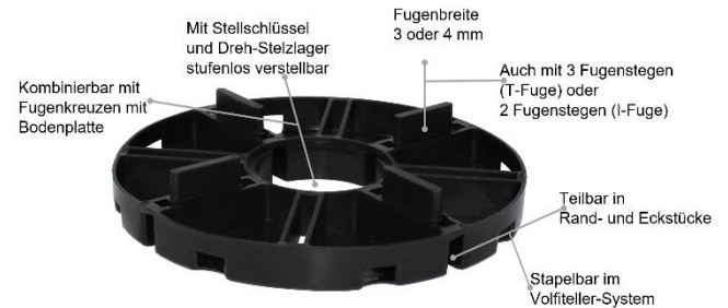
Abbildung 1: Volfiteller VT-B mit 4/10er Fuge 15mm hoch; 140mm Durchmesser.
