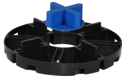
Abbildung 6: Ein FK-B mit größerer Fuge als der vorliegende VT-B versenkt sich in der mittigen Aussparung und hebt die Fuge des VT-B auf.
