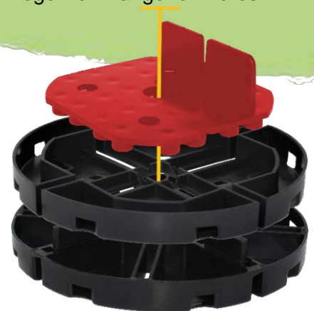
Abbildung 8: VT-B mit aufgesetztem Kombiteller und eingelegtem Volfilager. Das rote Element ist dabei nach Belieben austauschbar. Nutzen Sie so über 60 Fugenvariationen der Volfilager auch im Teller-System.
