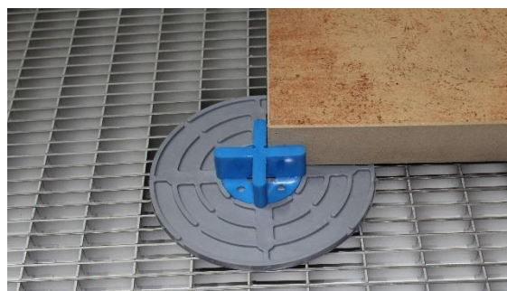
Abbildung 5: FK-B eingelegt in VP-GKU zur Verlegung auf Gitterrosten
